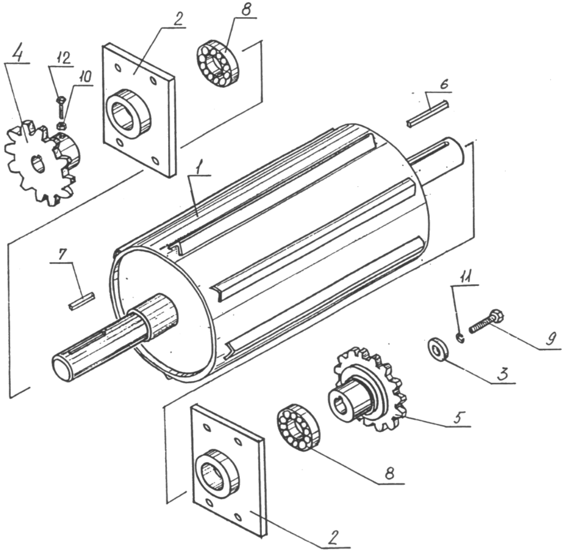
Рис.5 Барабан верхний ПРС 27.000 (рис.6)
