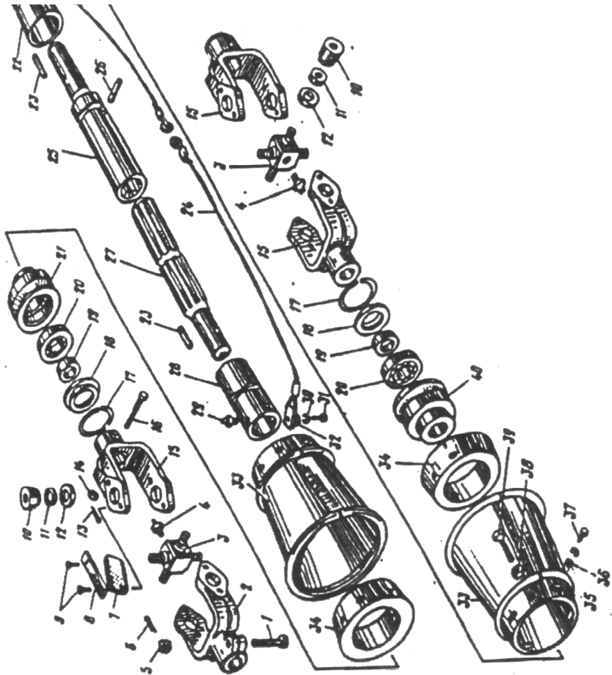
Вал промежуточный ЛКВ54.000 (рис.16)
