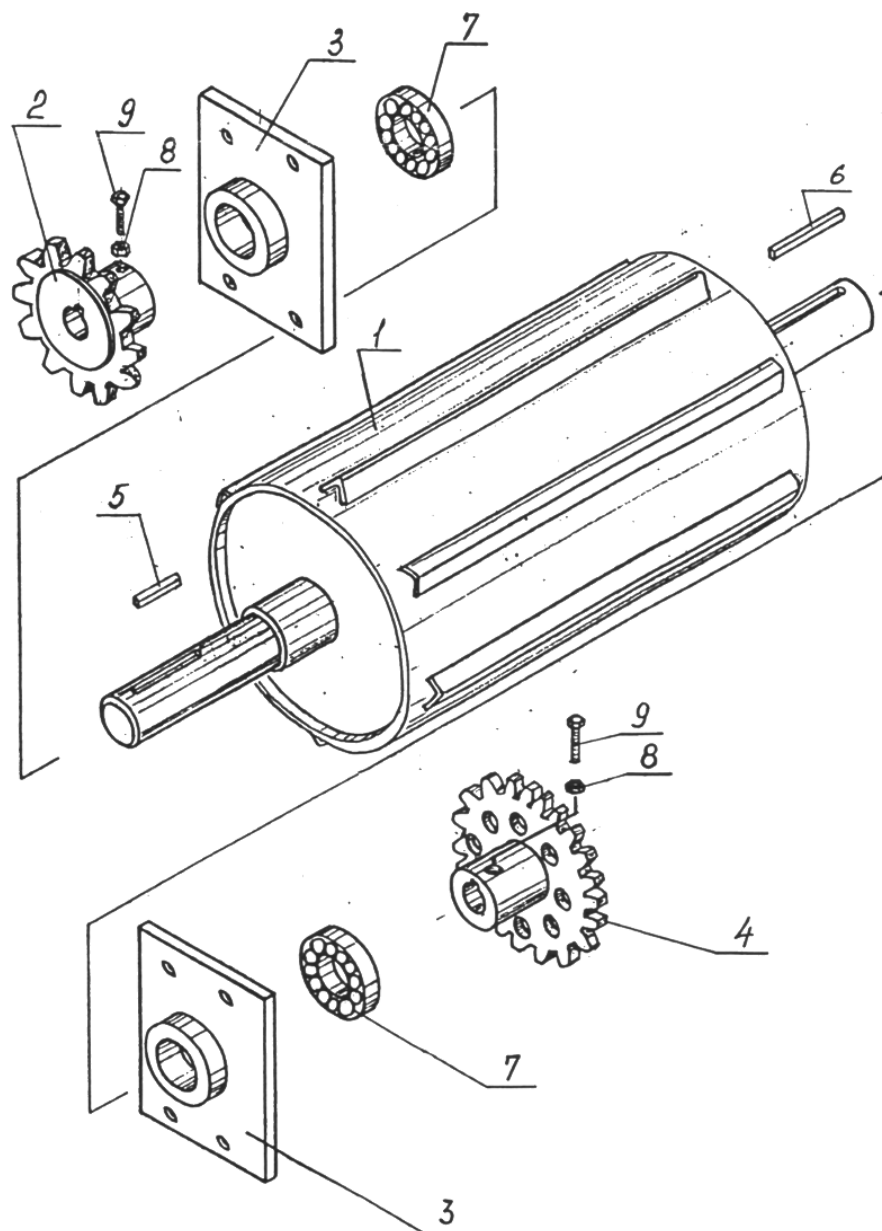
Рис.6 Подборщик ПРС 21.000( рис.7)
